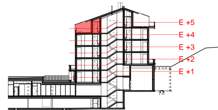
Schnitt Haus 2
